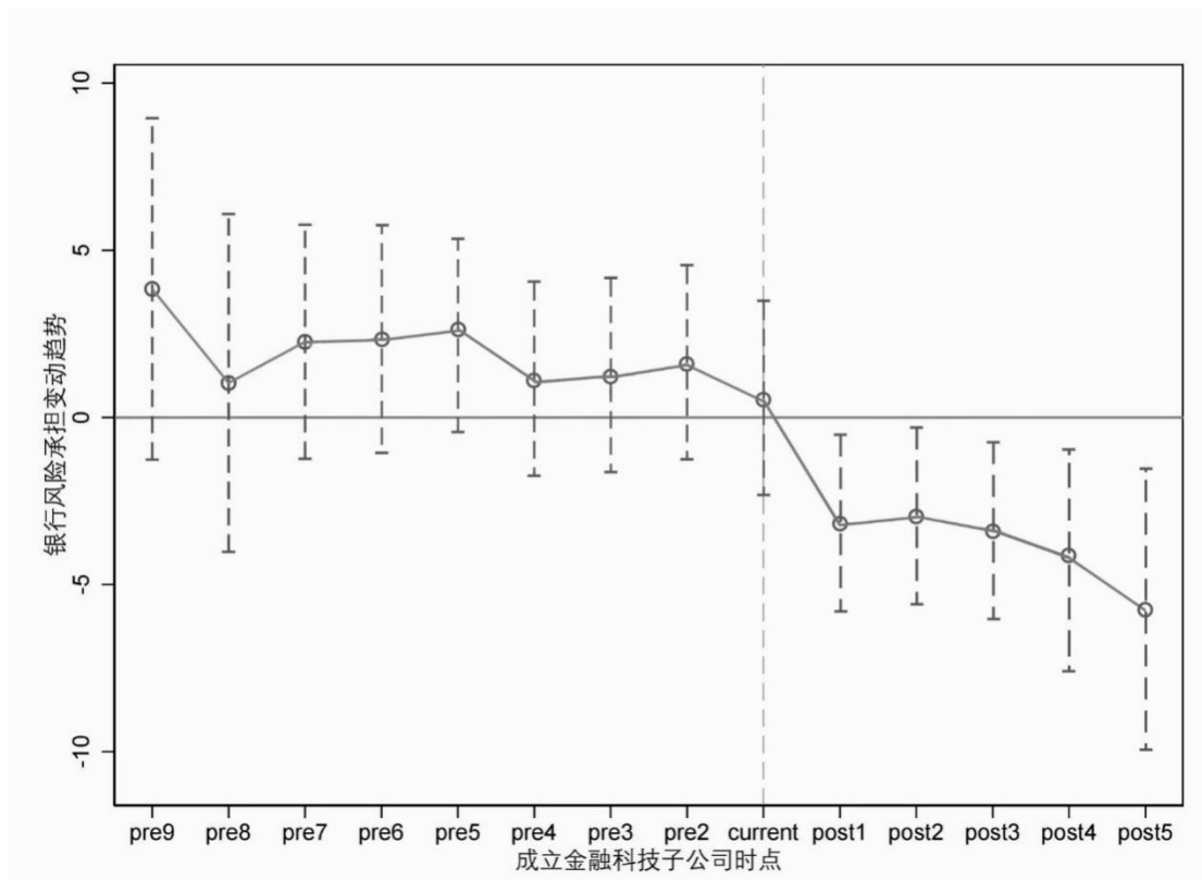
附图 2 平行趋势检验图
